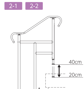
あがりかまち高さ20~40cm対応
